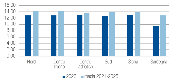
Proteine [% s.s.]
