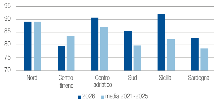
Altezza [cm]
