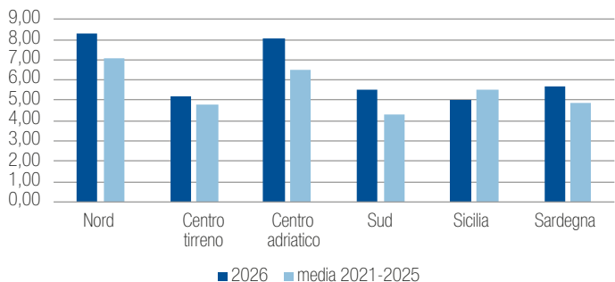
Produzione [t/ha]
