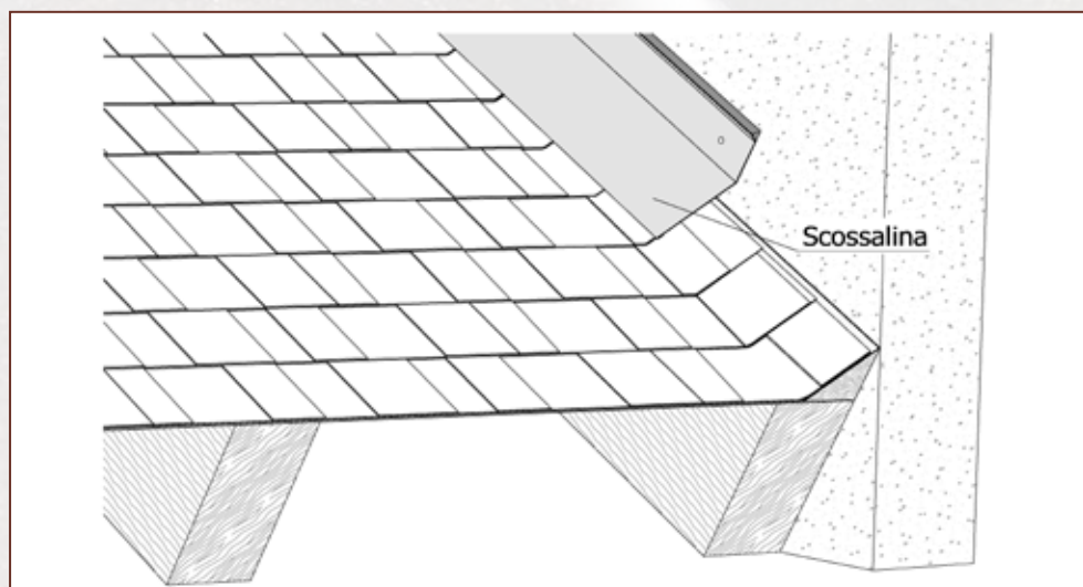
DETTAGLIO DI BORDO TETTO (figura 12)
