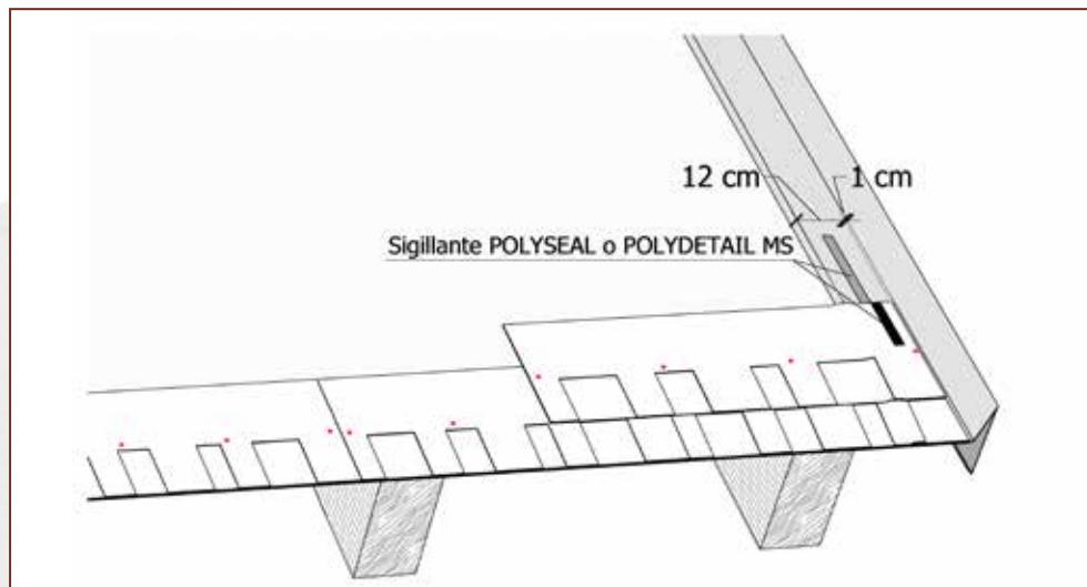
DETTAGLIO DI BORDO TETTO (figura 10)
