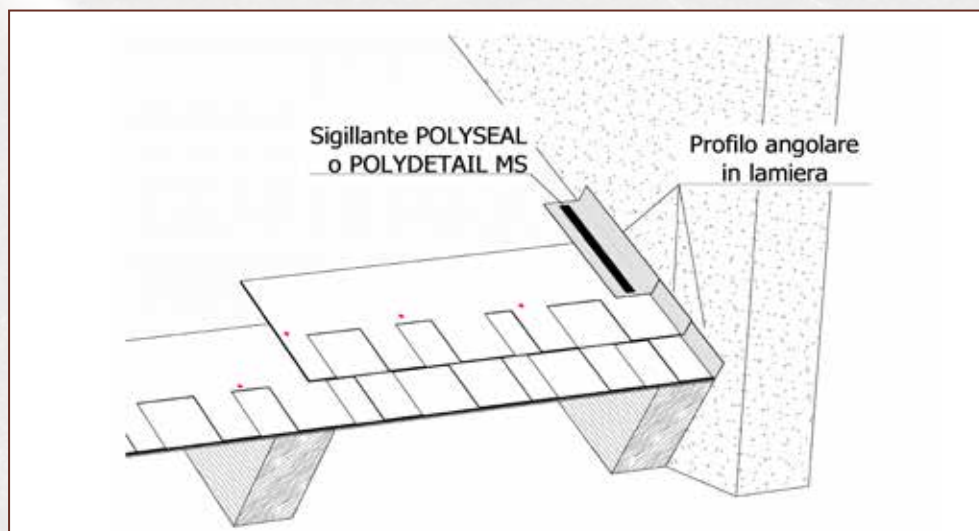
DETTAGLIO DI BORDO TETTO (figura 11)
