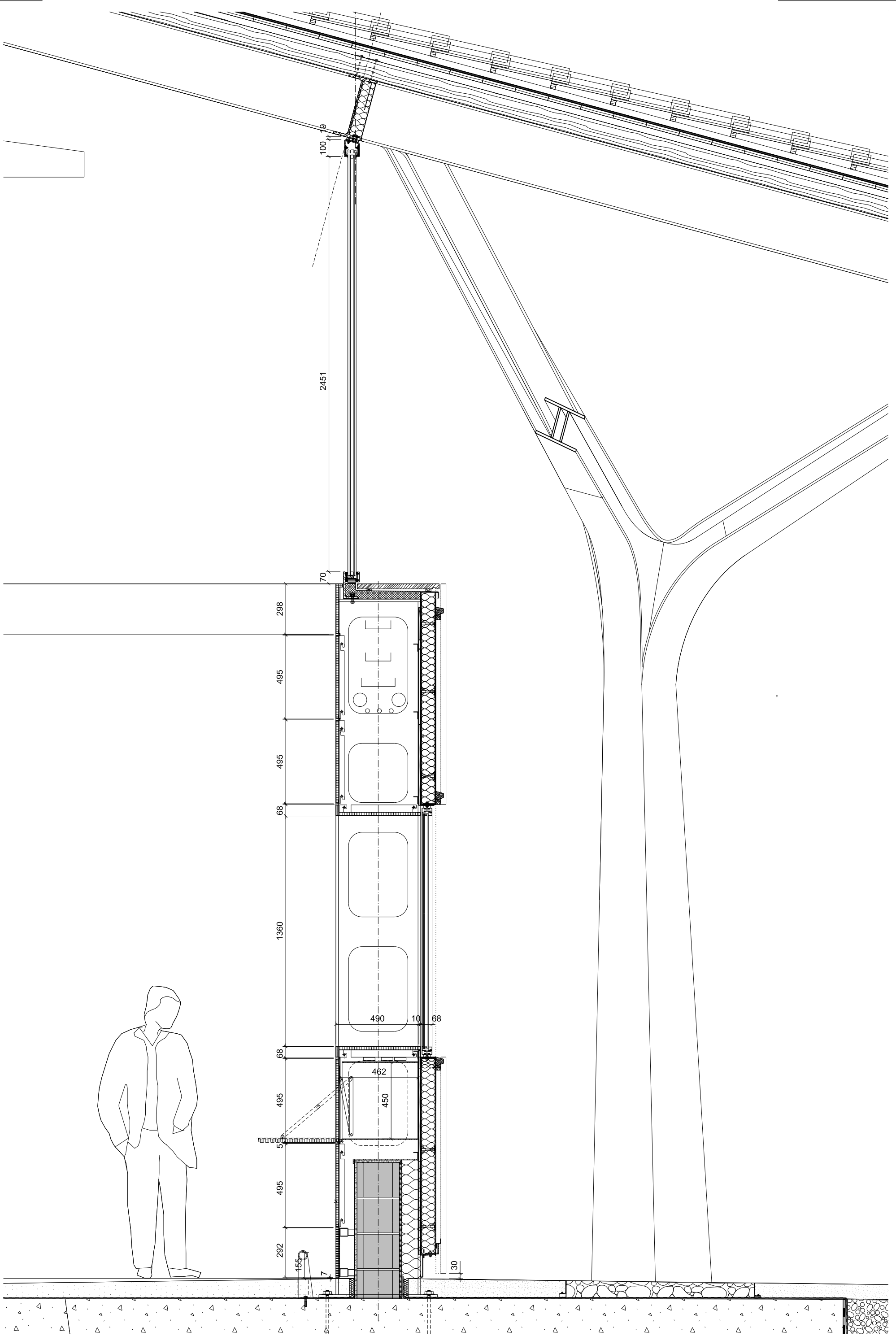
06e Coupe type du mur technique, avec unité de paillese
