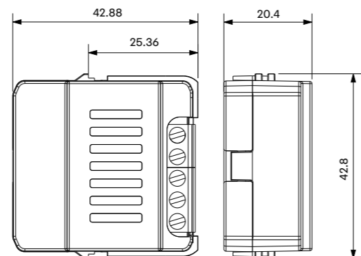
GW A1 918 Misuratore di energia connesso
