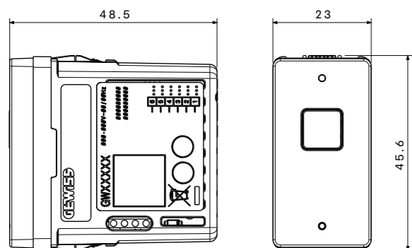
GWC 20 859 - GWC 21 859 - GWC 22 859 Attuatori 1 canale on/off connessi
