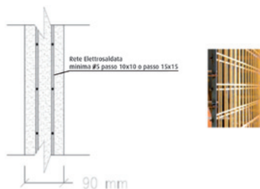
Figura 1.15: Rete elettrosaldata della parete della cabina
