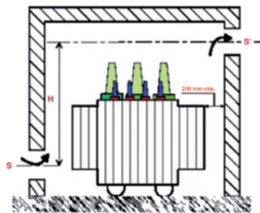
Figura 1.5: Aperture di ventilazione per ricambio d'aria naturale
