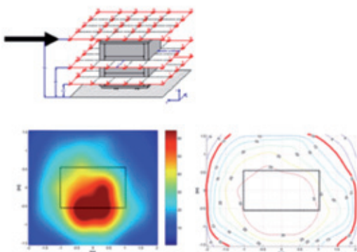
Figura 3.6: Andamento dell'induzione elettromagnetica in corrispondenza dell'attacco del condotto sbarre. il quadrato tratteggiato indica il box trasformatore
