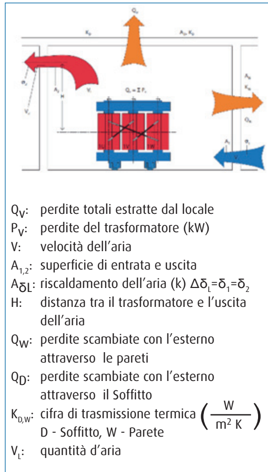
Figura 8.4: Esempio di calcolo della ventilazione naturale di un trasformatore
