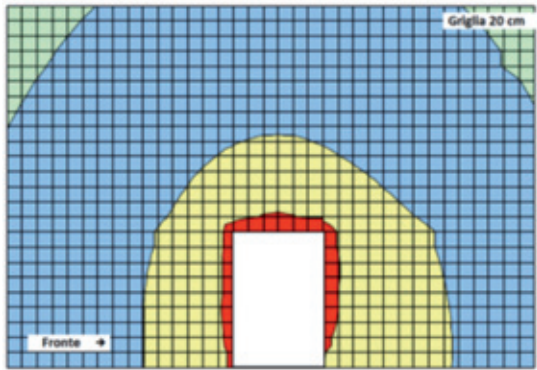
Figura 5.8: Rappresentazione grafica del campo magnetico (caso peggiore) intorno al QMT, visto dal lato (il fronte è a sinistra)
