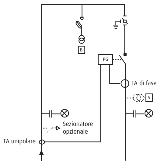
Figura 5.9: Schema con prescrizioni minime CEI 0-16
