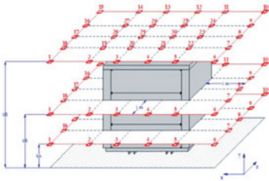
Figura 3.3: Piani di misura operazione per almeno altri 3 piani orizzontali.
