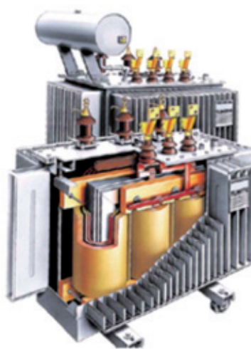
Figura 8.1: Trasformatore isolato in olio
