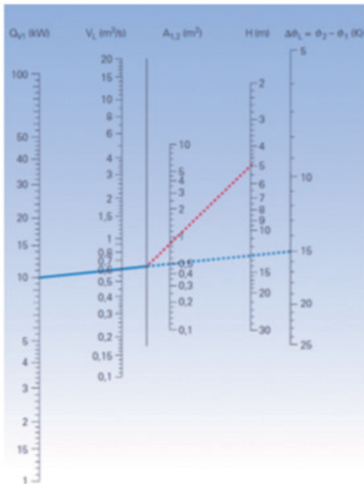
Figura 8.5: Grafico per valutazione ventilazione
