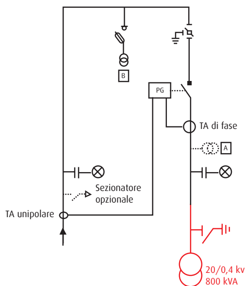
Figura 5.10: Schema connessione con sezionatore di terra lato carico
