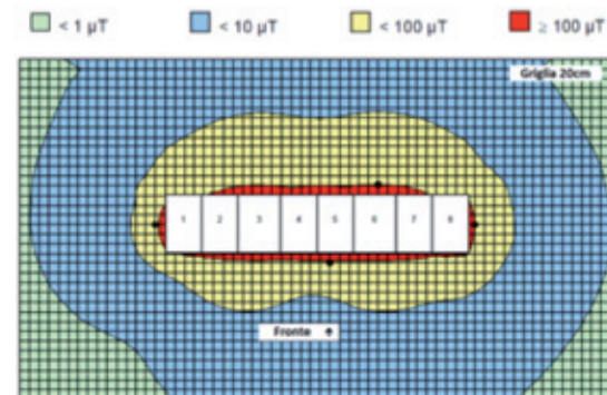
Figura 5.6: Rappresentazione grafica del campo magnetico (caso peggiore) intorno al QMT, visto dall'alto
