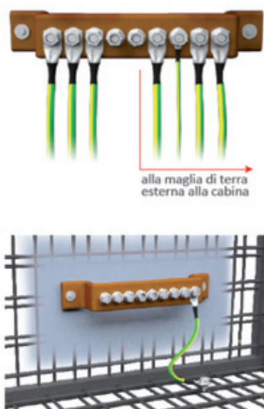
Figura 1.17: Collegamento impianto di terra
