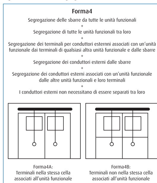
Figura 6.1: Forma di segregazione 4
