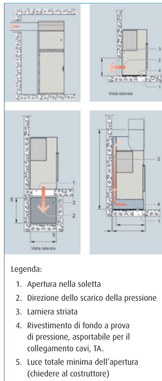
Figura 5.3: Sistema di canalizzazione della pressione verso l'esterno (1° immagine) o verso il retro (2° immagine) o verso il basso (3° immagine) o l'alto (4° immagine)
