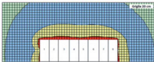
Figura 5.7: Rappresentazione grafica del campo magnetico (caso peggiore) intorno al QMT, visto dal fronte
