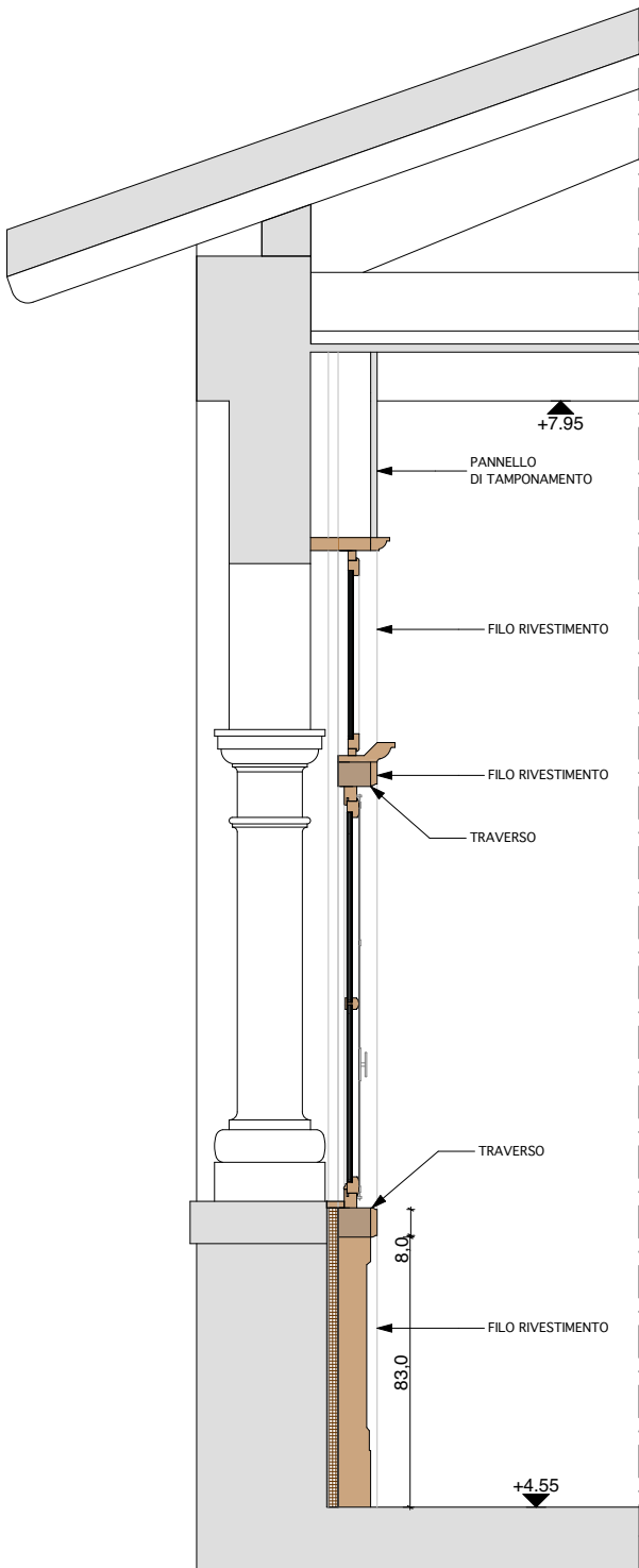
SEZIONE A-A
