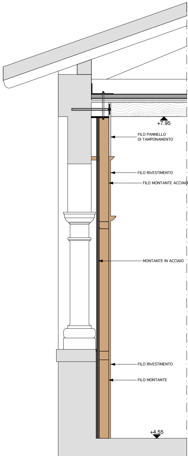
SEZIONE B-B
