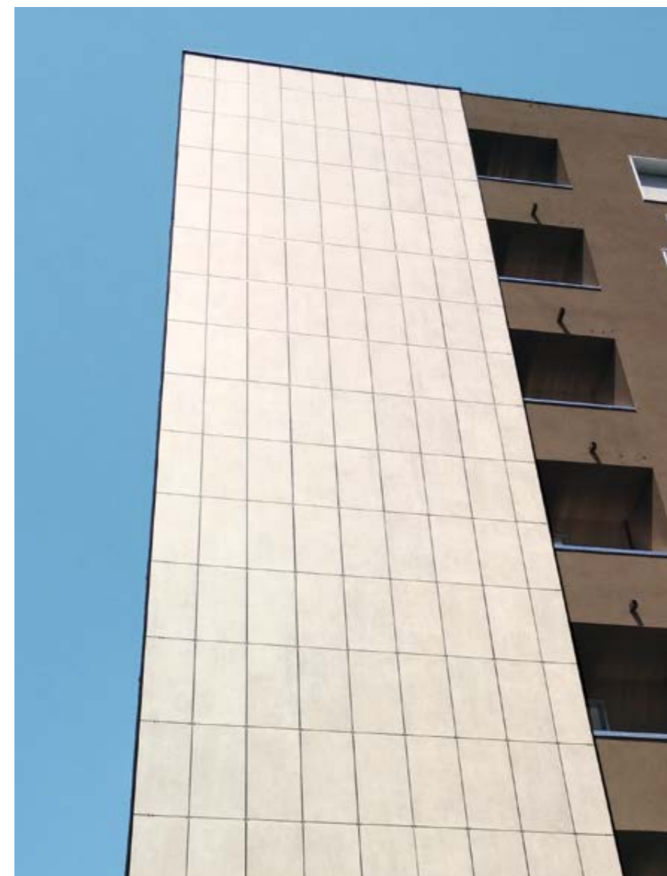
60x120 cm 60x120 cm FACCIATA ISOLATA VENTILATA VENTILATED INSULATED FACADE SISTEMA DI AGGANCIO A VISTA VISIBLE ANCHOR SYSTEM
