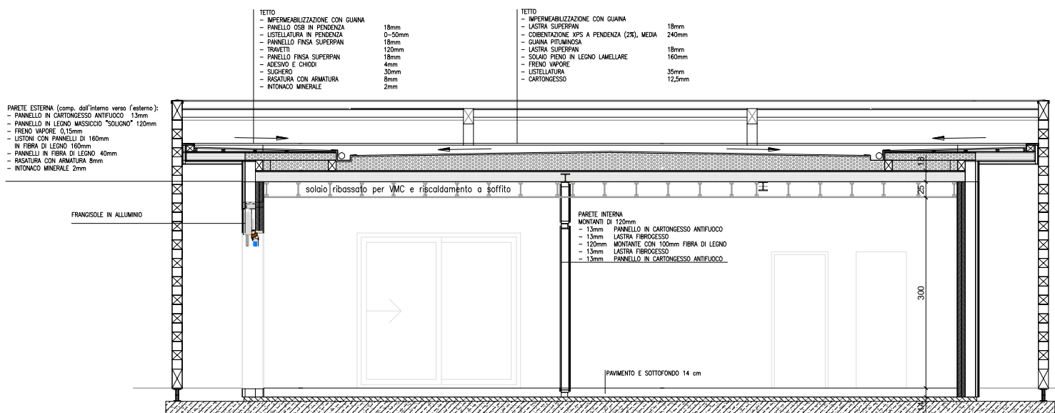
SEZIONE CON PARTICOLARI COSTRUTTIVI
