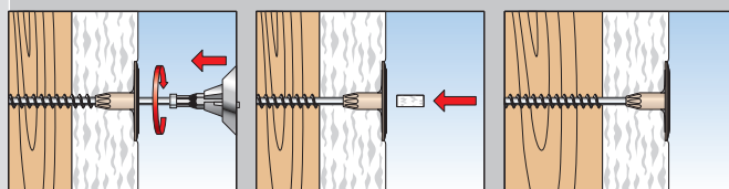
Sequenza per l'installazione di Termofix 6H-NT a filo dei pannelli isolanti
