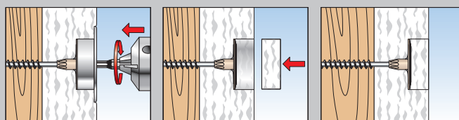
Sequenza per l'installazione di Termofix 6H-NT a scomparsa nei pannelli isolanti.
