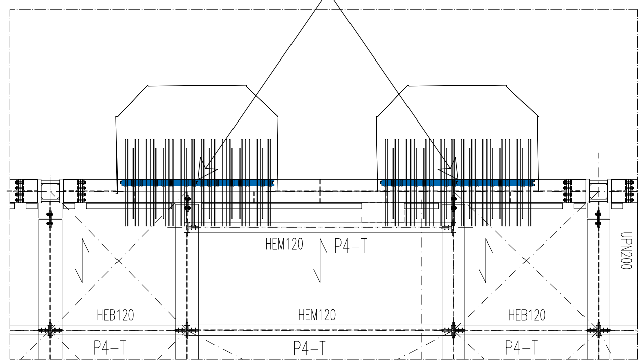
Schöck Isokorb tipo A-K 12/6-h160
