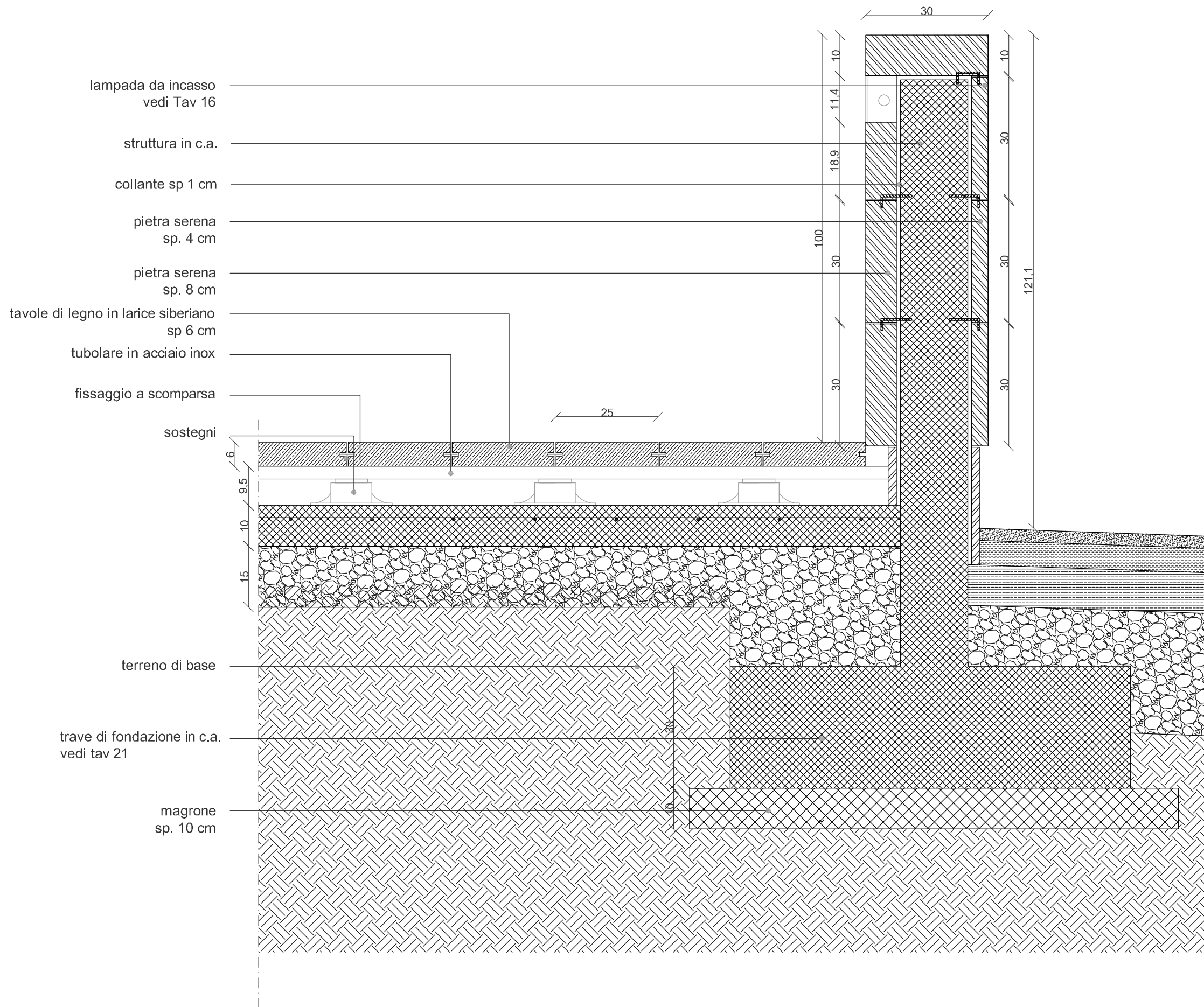
Sezione P-P'
