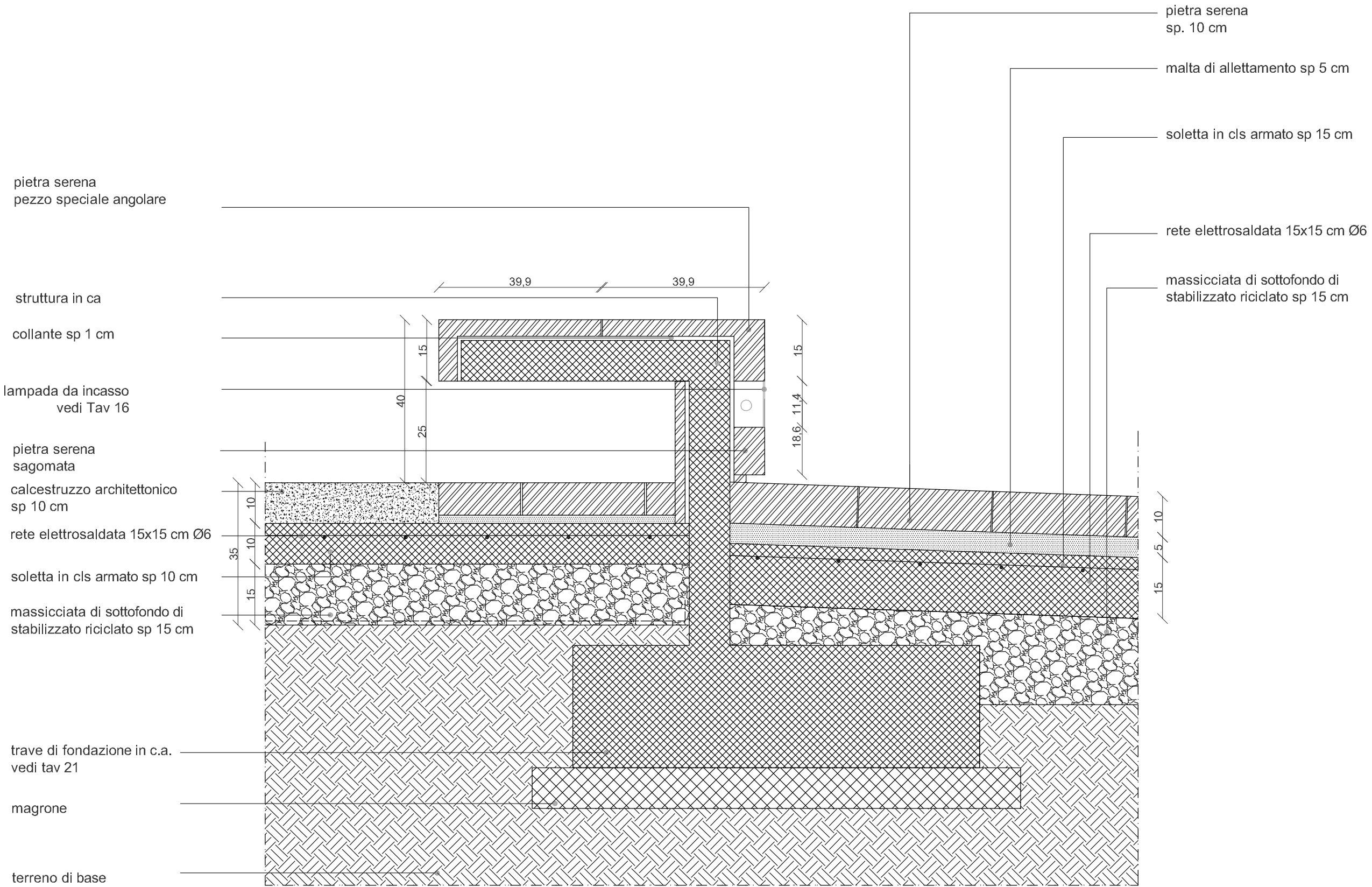
Sezione H-H'
