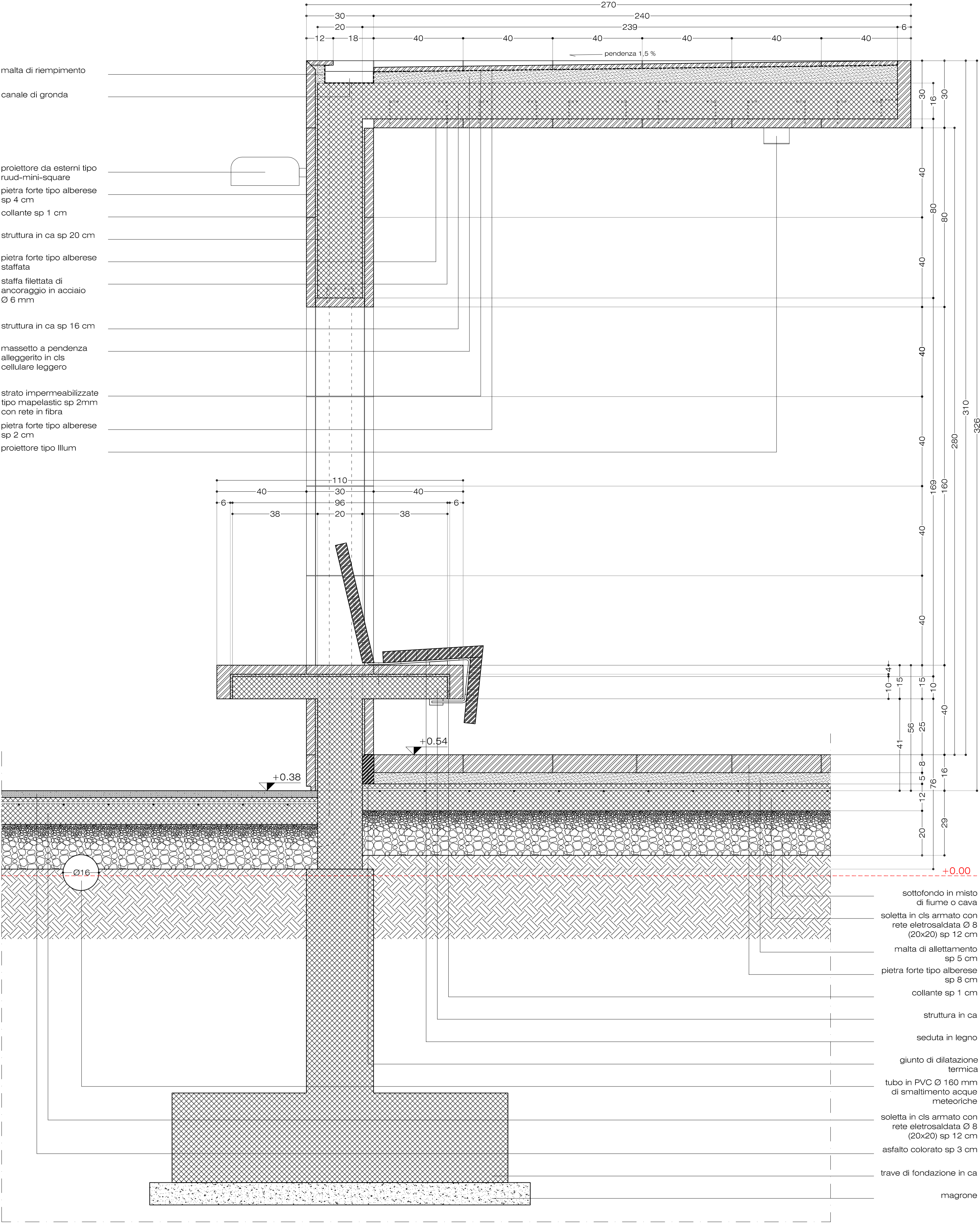
sezione 5-5
